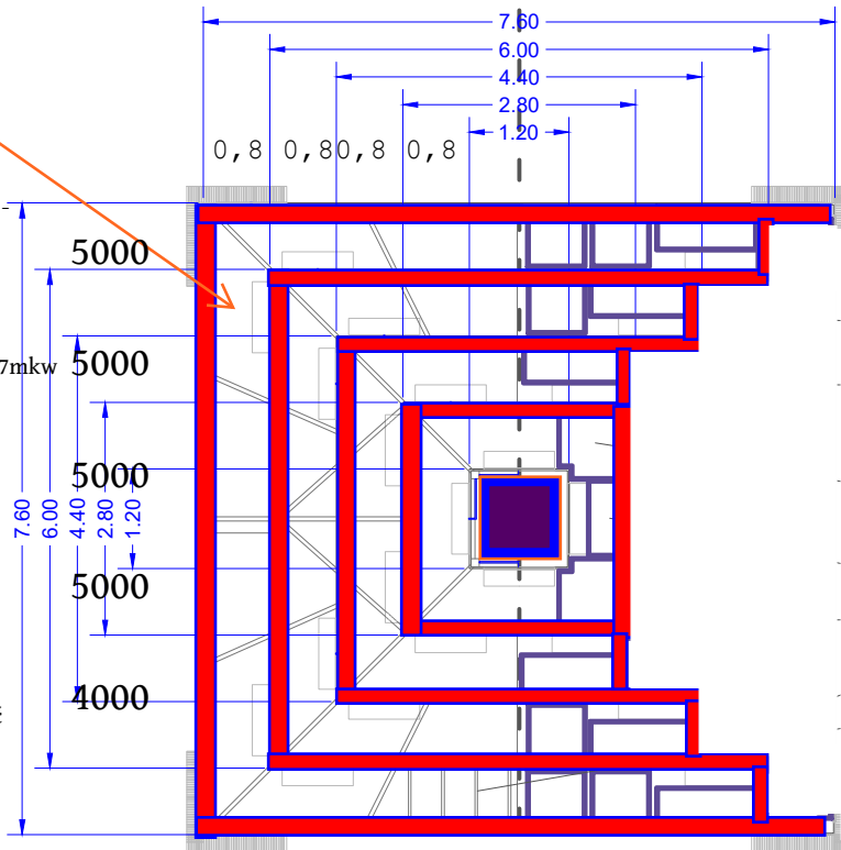
Rzut konstrukcja stalowa:
